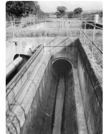
Stauschild, Patent EP 0509422
